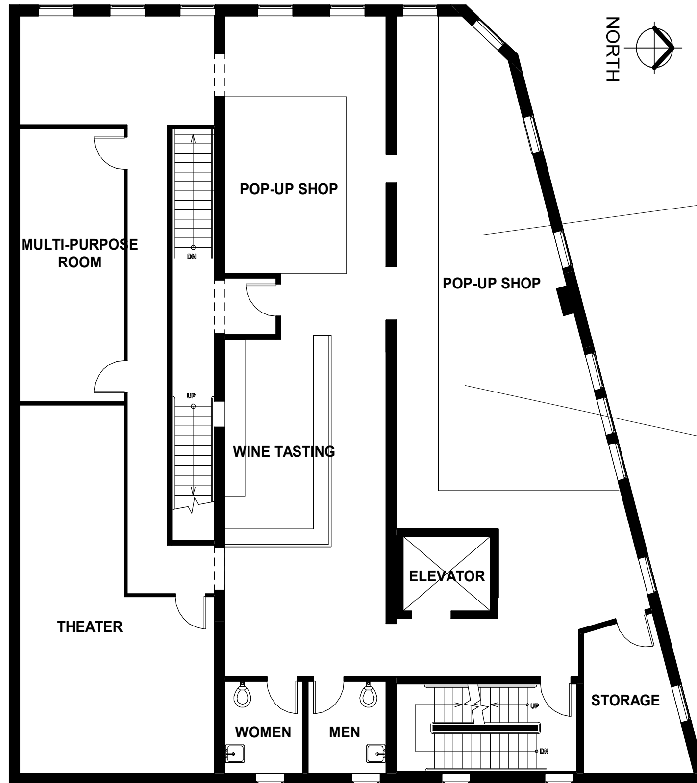
► FLOOR PLAN
